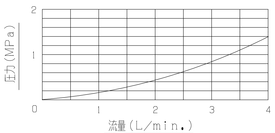
圧力降下特性 (弁全開時)
