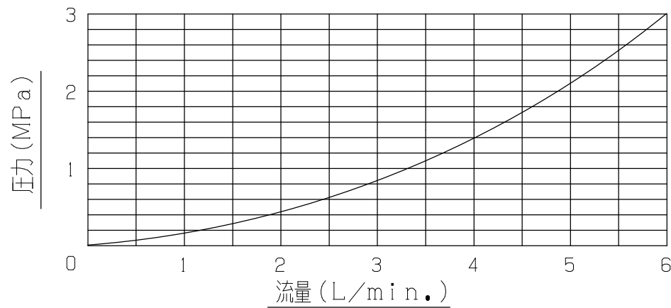
圧力降下特性 (弁全開時)
